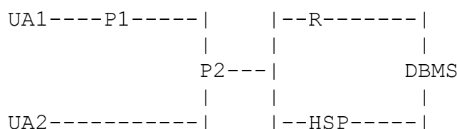
Рис 2.2. Пример сети, использующей заголовок Service-Route
