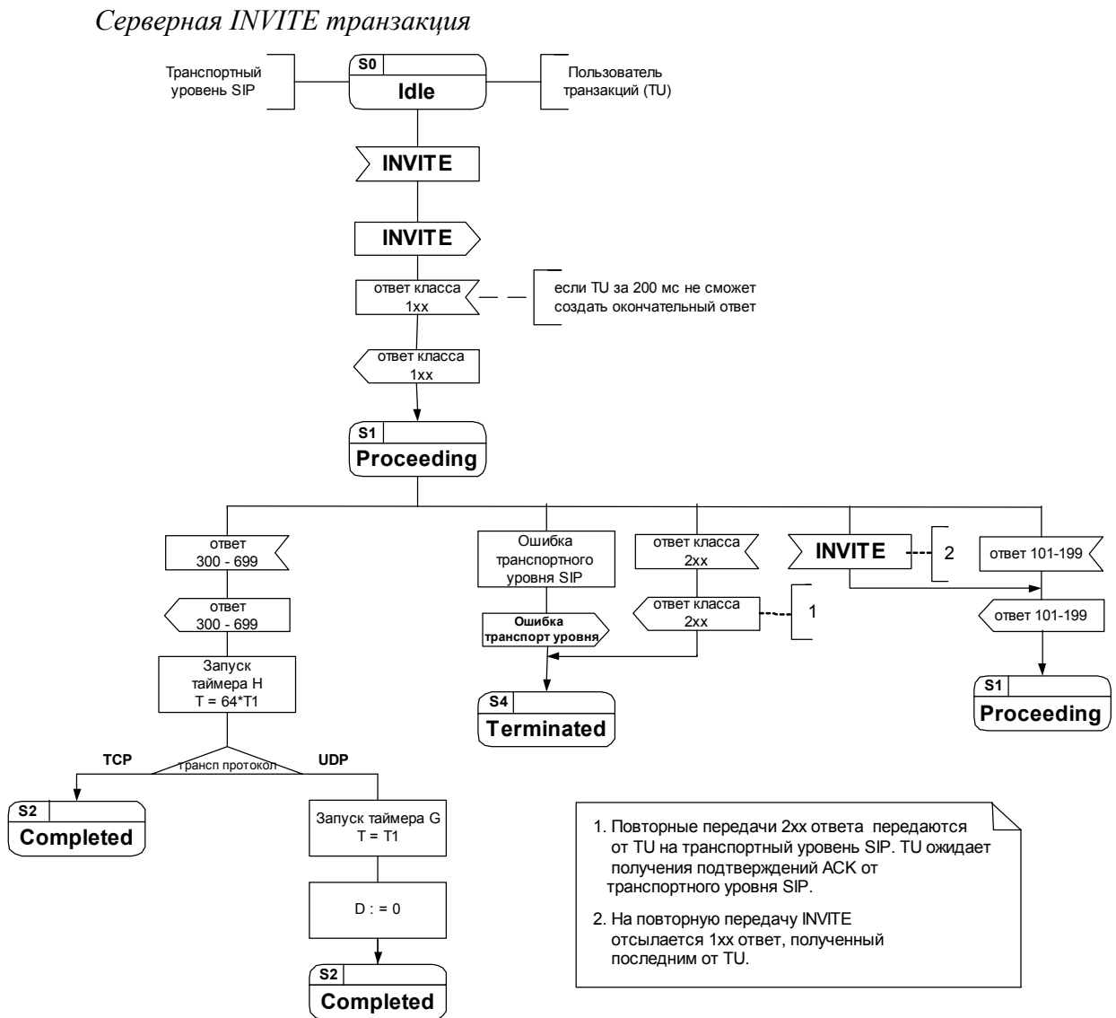
Рис.2.24. Переход в состояние Proceeding.
