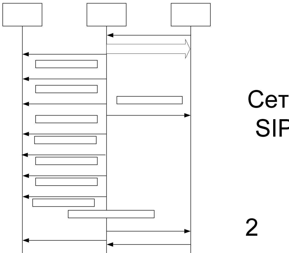
Рисунок 3.9 Диаграмма обмена сообщениями при истечении таймеров в сети SIP.
