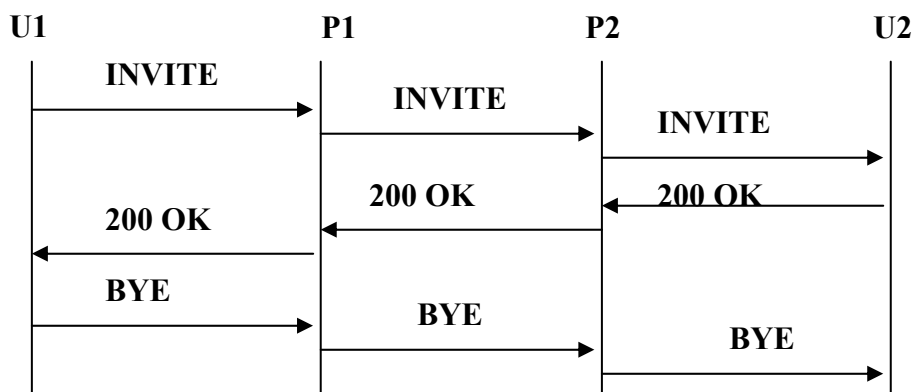
Рис. 2.35. Взаимодействие через исходящий и входящий прокси-серверы
