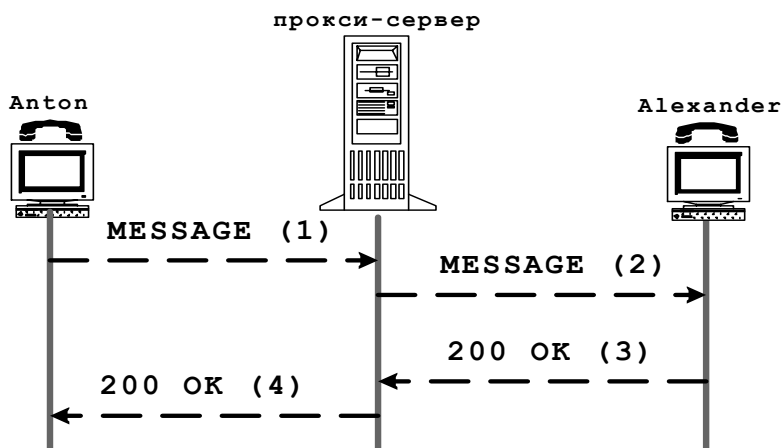
Рис. 2.9 Пример использования запроса MESSAGE
