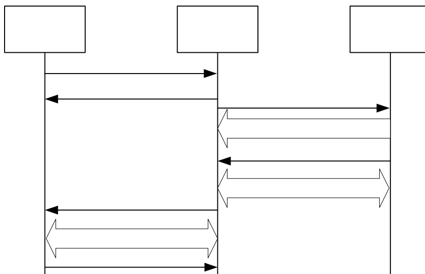
Рисунок 3.30 Диаграмма обмена сообщениями при успешном установлении соединения SIP – ТфОП. Используется быстрый ответ.
