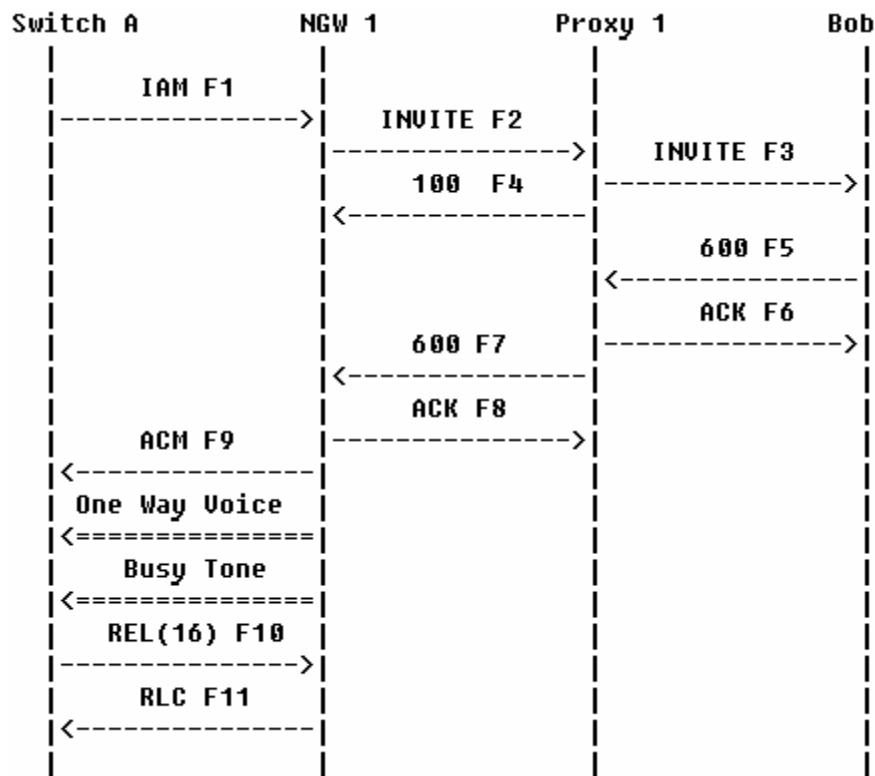
Рисунок 3.25 Диаграмма обмена сообщениями при неуспешном установлении соединения ТфОП – SIP. Линия занята. IAM содержит параметр interworking.
