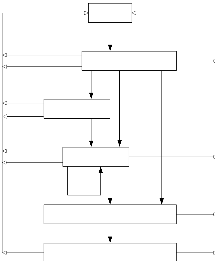
Рисунок 3.36 Конечные автоматы SIP-T при взаимодействии SIP-ISUP.
