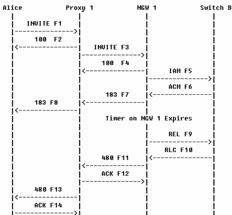
Рисунок 3.49 Диаграмма обмена сообщениями. Неуспешное установление соединения SIP – ТфОП. Истекает таймер ожидания сообщения ANM.
