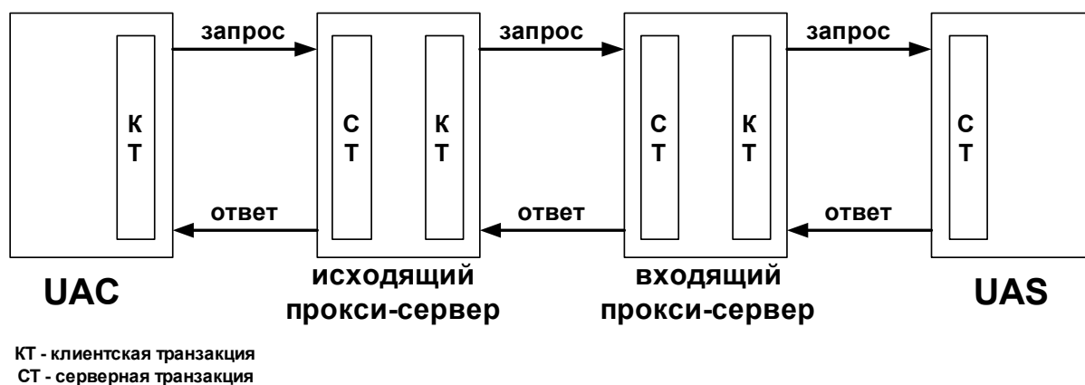
Рис 2.11 Взаимодействие клиентских и серверных транзакций.
