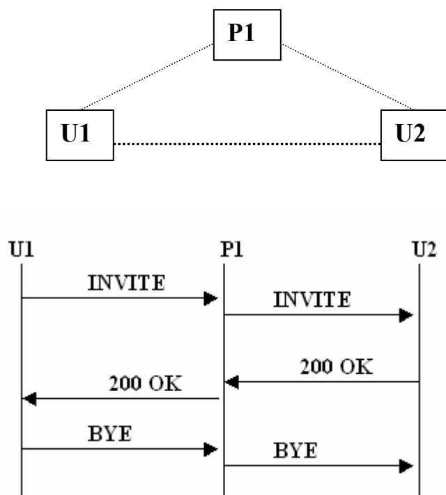
Рис. 2.37 Прохождение сообщений через прокси-сервер с перезаписью значения в заголовке Record-Route
