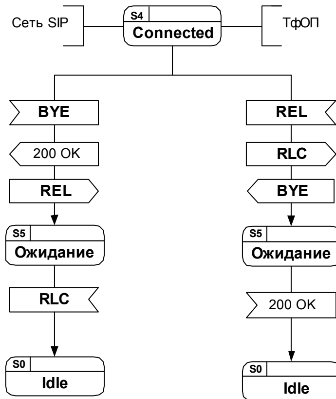
рисунки 3.19 Переходы из состояния «Connected»
