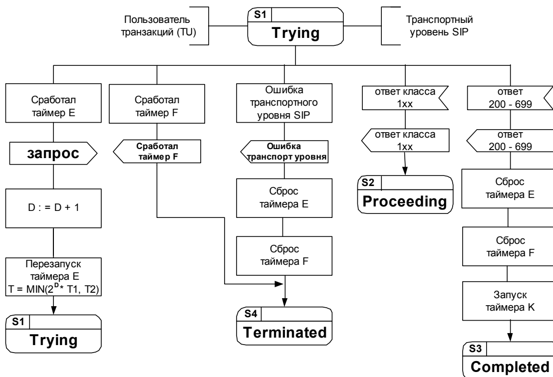
Рис.2.20. Переход в состояние Trying.
