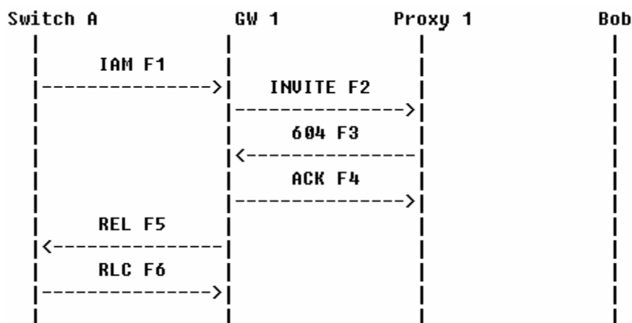
Рисунок 3.23 Диаграмма обмена сообщениями при неуспешном установлении соединения ТфОП – SIP. Пользователь не найден.
