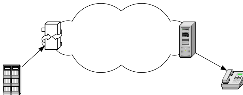
Рисунок 3.3 Сеть в случае установления соединения ТфОП – VoIP.
