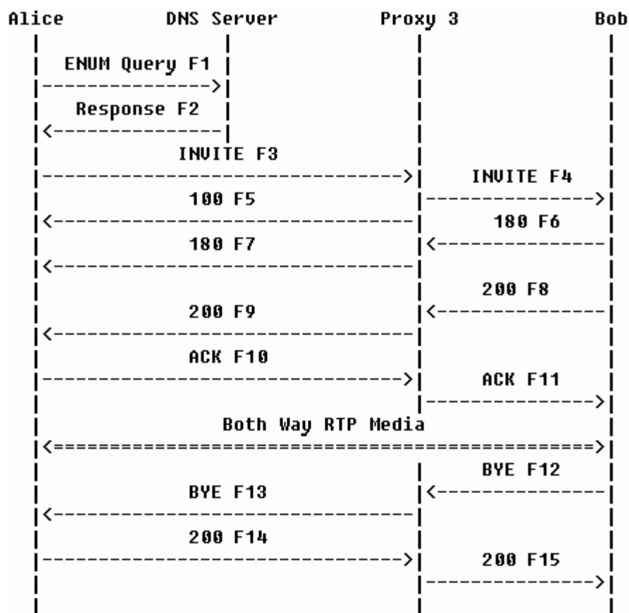
Рисунок 3.46 Диаграмма обмена сообщениями. Успешное установление соединения внутри сети SIP с использованием ENUM Query.
