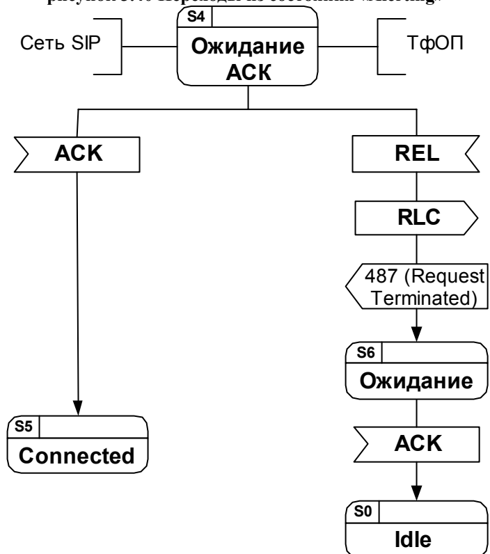
рисунок 3.41 Переходы из состояния «Ожидание ACK»
