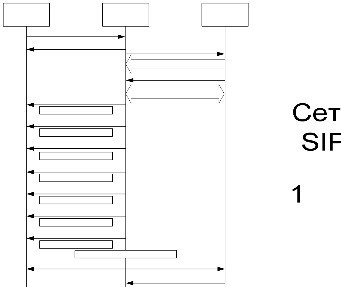
Рисунок 3.32 Диаграмма обмена сообщениями при истечении таймера T1 сети SIP.
