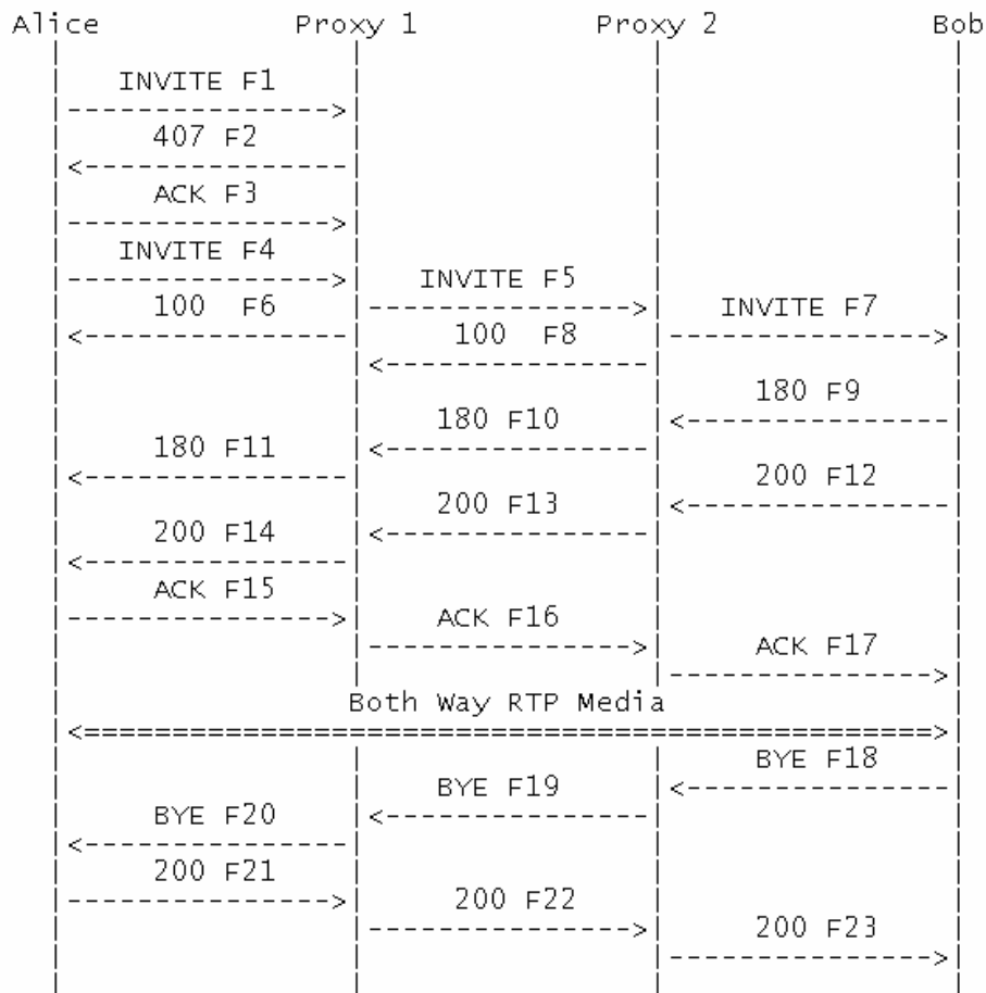
Рис. 2.39 Установление соединения с участием прокси-серверов
