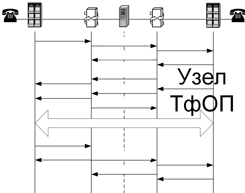
Рисунок 3.2 Пример обмена сообщениями между узлами ТфОП при транзите трафика через сеть VoIP.
