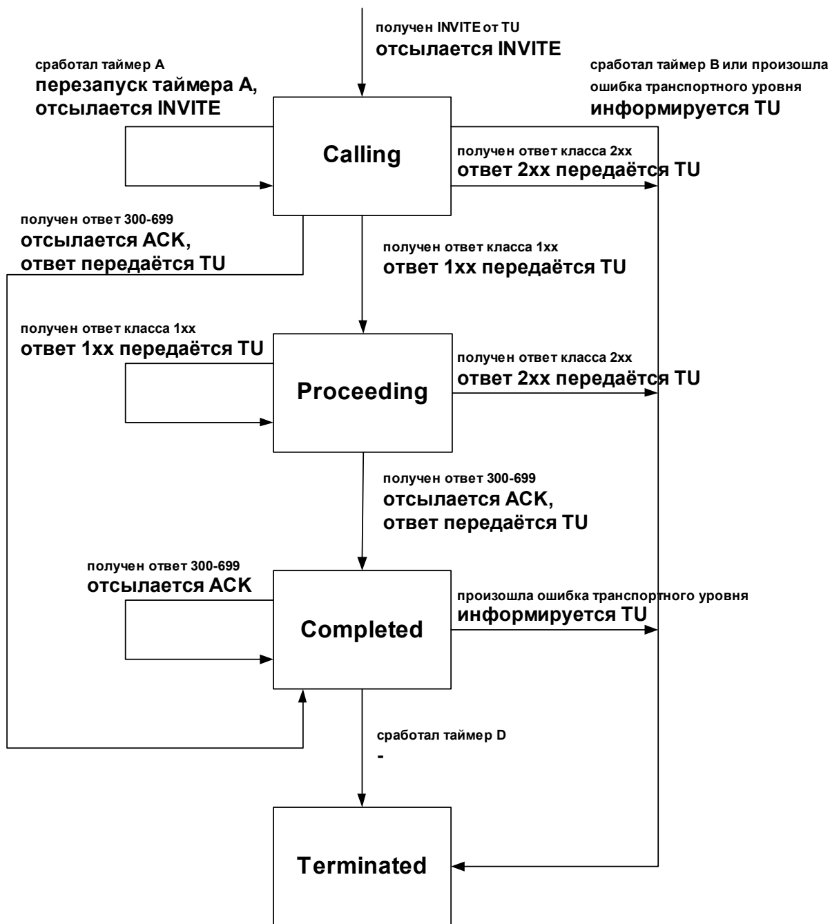
Рис. 2.12 Клиентская INVITE-транзакция.
