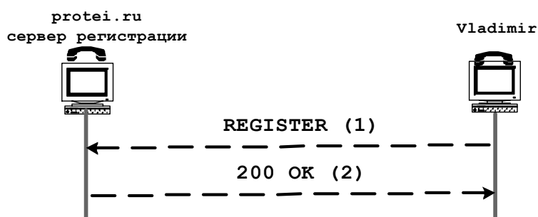
Рис. 2.31 Процедура регистрации
