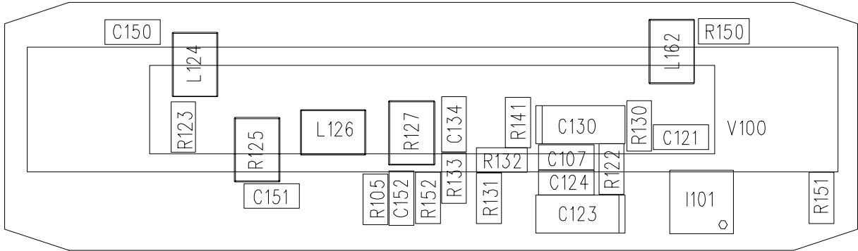
The Top Side Layout PO0313
