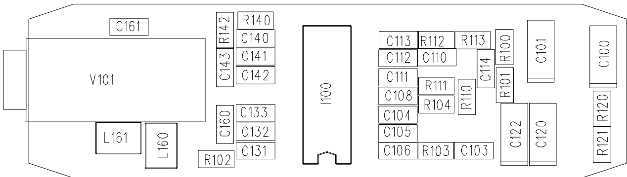
The Bottom Side Layout PO0313
