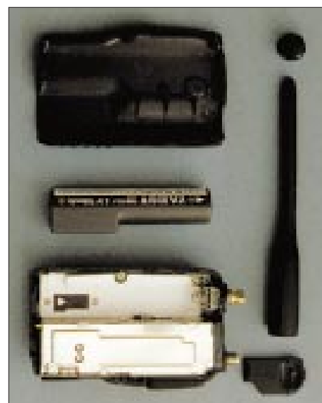
Das zerlegte VX-1R. In der Mitte ist der Lithium-Ionen-Akku, der etwas größer als eine Mignonzelle ist. Fotos: FA
